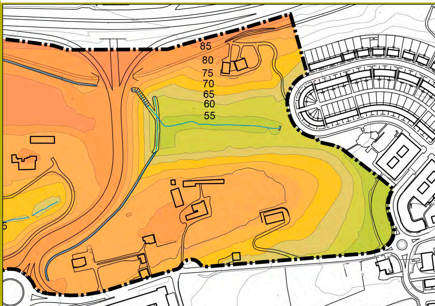
Lekungo parajearen plano hipsometrikoa. Argi eta garbi ikusten dira desnibel handiak.
